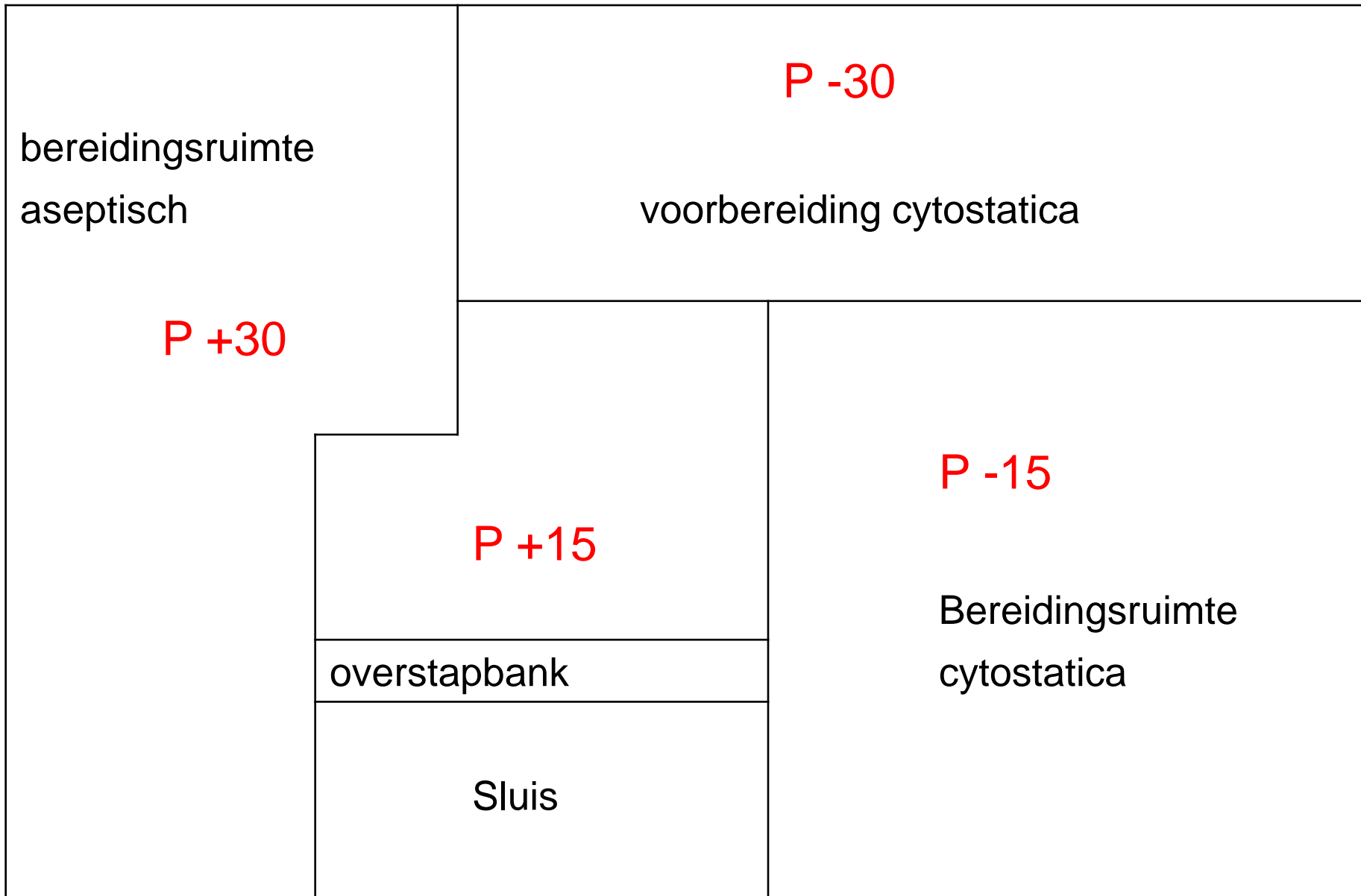
Schematisch de bereidingsruimten incl. drukhierarchy
